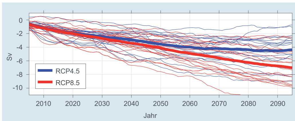
Abbildung 8: Die mit verschiedenen Klimamodellen für das 21. Jahrhundert projizierte und mit einem Zehn-Jahre-Filter geglättete Änderung der Umwältzirkulation (Sv) bei 30^\circ N gegenüber 1970-2000, deren Ergebnisse im 5. Sachstandsbericht des Weltklimarats Eingang gefunden haben. Gezeigt sind Ergebnisse für zwei Treibhausgasszenarien: Ein moderates Szenario (RCP4.5, blaue Linien) und ein „Worst-Case-Szenario“ (RCP8.5, rote Linien). Das RCP8.5 Szenario entspricht einer äquivalenten \text{CO}_2 -Konzentration von 1370 ppm (parts per million) gegen Ende des 21. Jahrhunderts gegenüber 650 ppm im RCP4.5 Szenario. Die Mittelwerte über alle Modelle sind als fette Linien gezeigt. Die Stärke der Umwältzirkulation bei 26,5^\circ N im Zeitraum 1970-2000 beträgt im Mittel über alle Modelle 19 Sv. Die gemessene Stärke bei 26,5^\circ N lag von April 2004 bis Oktober 2015 bei 16,9 \pm 4,4 Sv.
